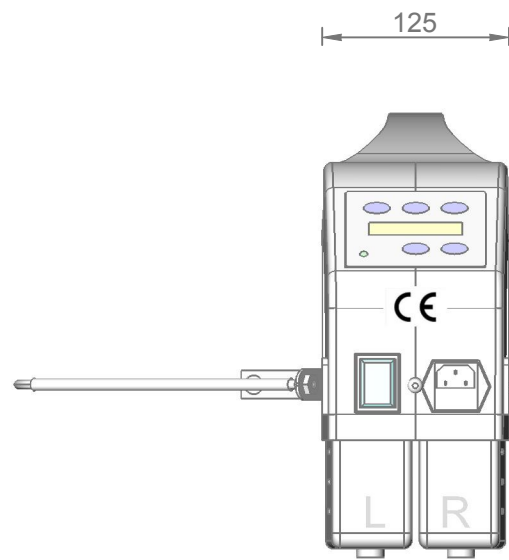
invoerzijde (bedieningspaneelzijde)
