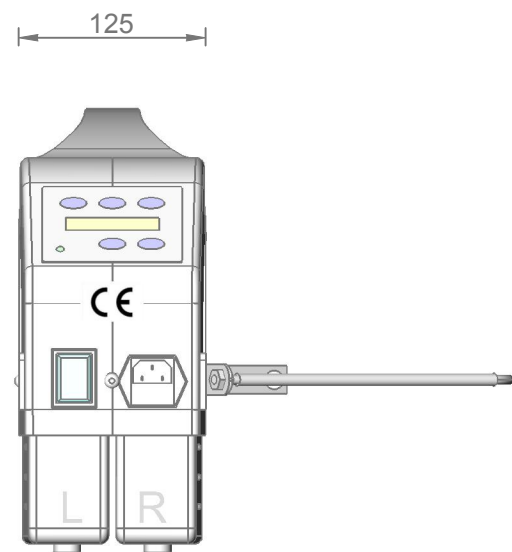
invoerszijde (bedieningspaneelzijde)
